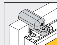
Klämfäste (för montage på fönsterbåge där man ej vill borra, t.ex. PVC-fönster) L1, L3, FS1, FS2, FS3, M1, K4
